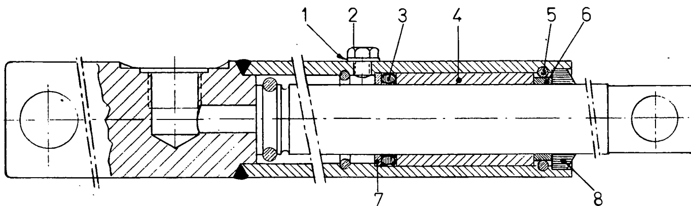
HEFCILINDER - CYLINDER - VERIN - ARBEITSZYLINDER 330893
